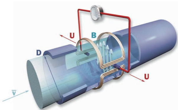
图 1 工作原理图
