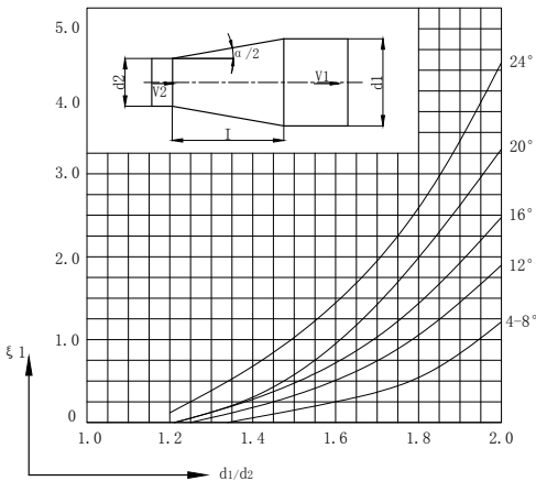
渐扩管
