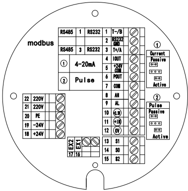
图 5 一体式接线图
